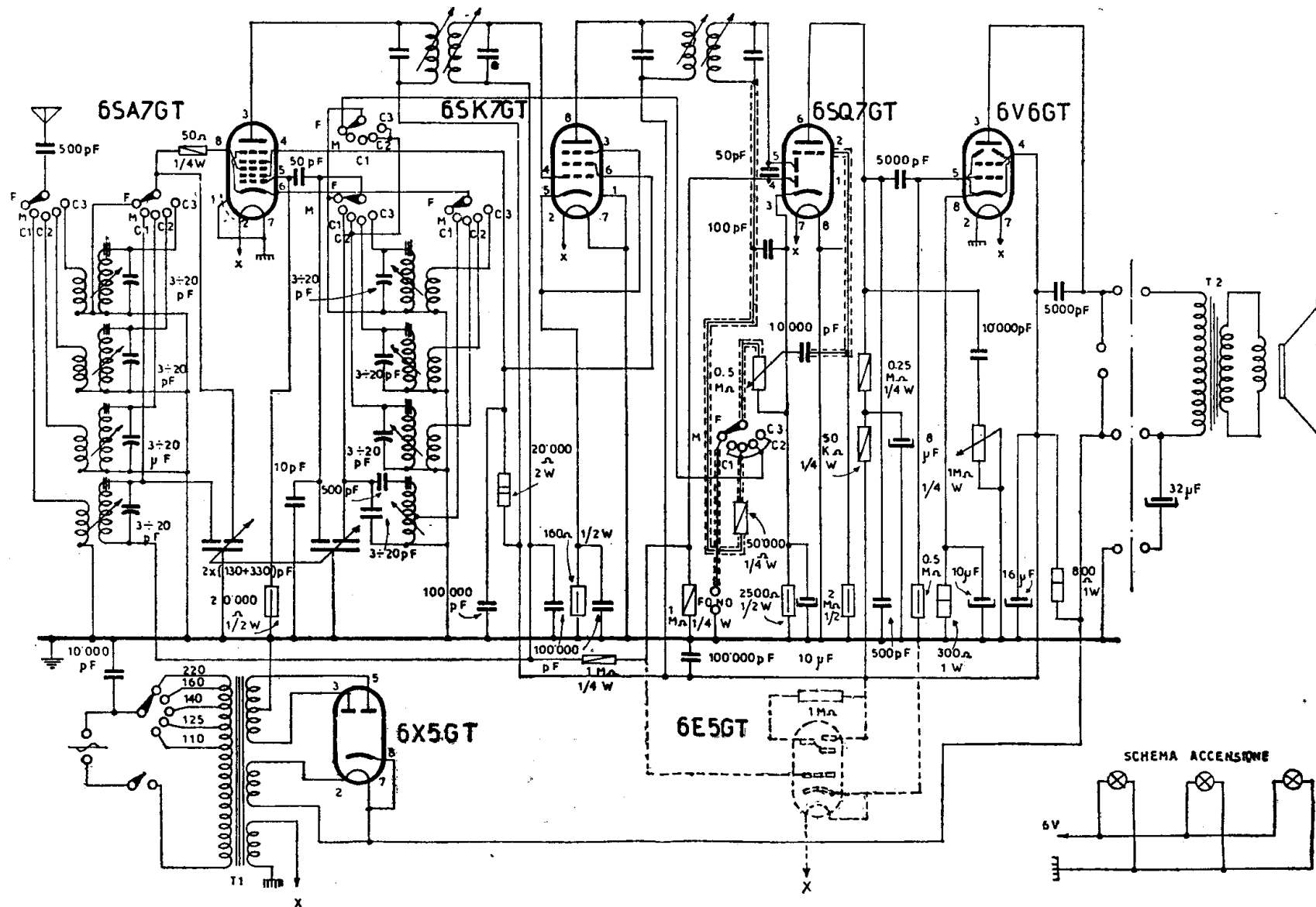
DUCATI SSR - Modd. 4160, 4250 e 4260 - Il mod. 4160 con occhio magico, il 4260 con occhio magico ed espansore di gamma. MF a 462 kc. Placca finale 250 V.
